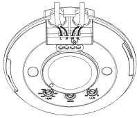
Przewody wychodzą z boku
