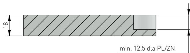
A-A (1 : 2)
