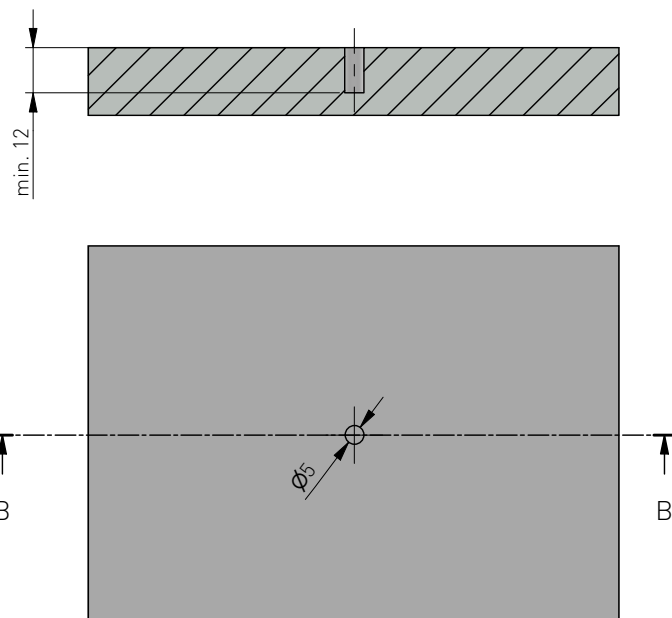
B-B (1 : 2)
