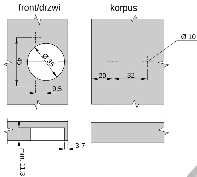
Wymiary montażowe / Mounting dimensions / Монтажные размеры
