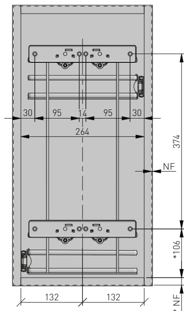
Wymiary produktu Product dimensions Размеры продукта
