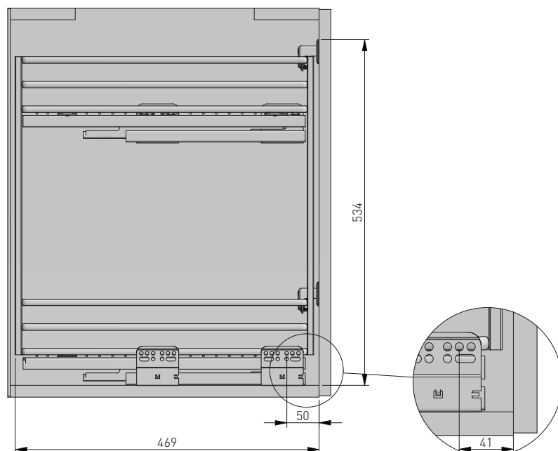
Rozstaw otworów montażowych w korpusie Spacing of mounting holes in the body Расстояние между монтажными отверстиями в корпусе
