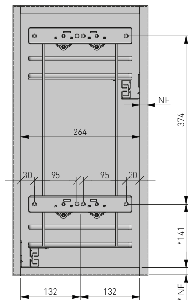
Wymiary produktu Product dimensions Размеры продукта
