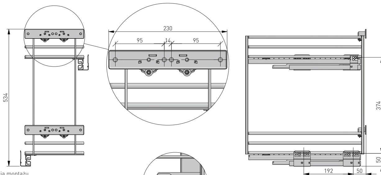
Proponycja montażu Installation proposal Предложение по установке
