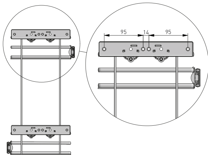
Proponycja montażu Installation proposal Предложение по установке
