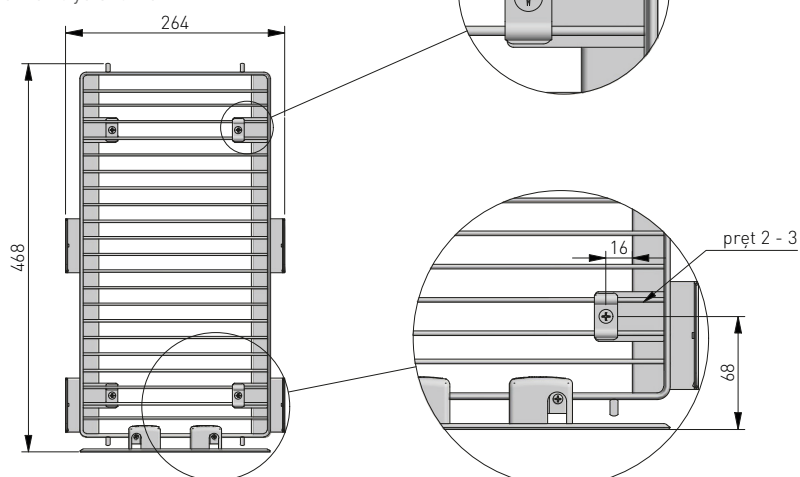
Proponycja montażu Installation proposal Предложение по установке
